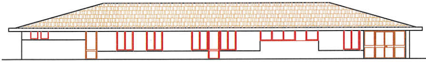
PROSPETTO OVEST
