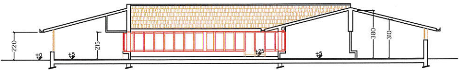
SEZIONE A-A
